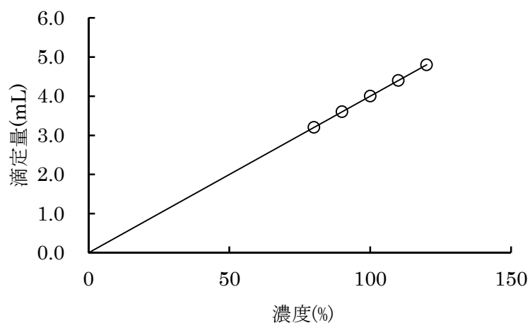
図*** 定量法 直線性
