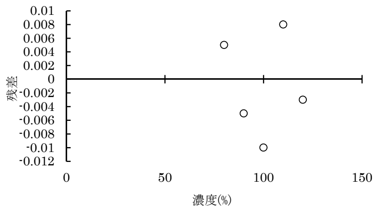
図*** (5) 定量法 残差プロット
