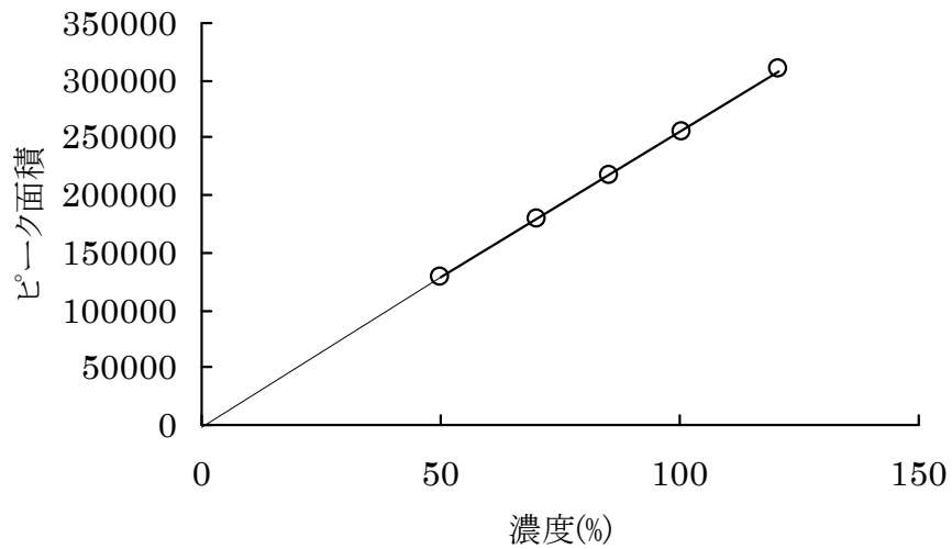
図*** (4) 溶出性 直線性
