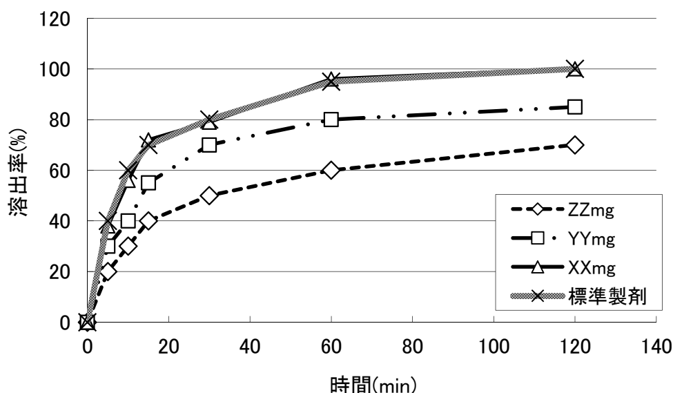
図*** 可溶化剤■■■の処方量と溶出挙動
